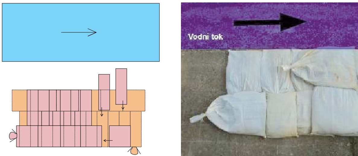
Obr. 10, 11 Kombinované víceřadé kladení jednokomorových pytlů
